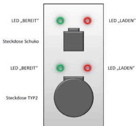
Abbildung - Bedienelemente Typ 2 Stecker (400 V, 16 A); Schuko Stecker (230 V, 16 A)
