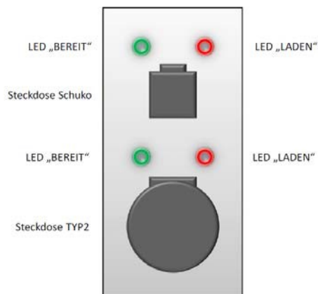
Abbildung - Bedienelemente Typ 2 Stecker (400 V, 16 A); Schuko Stecker (230 V, 16 A)
